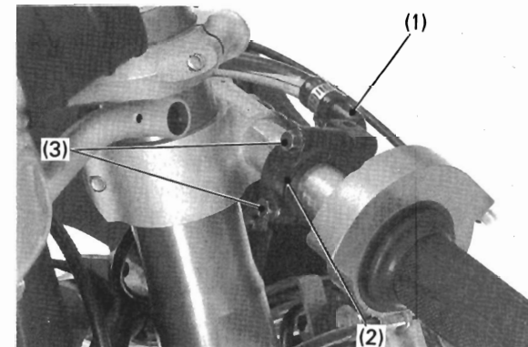
(1) マスタシリンダ (2) “UP”マーク (3) ボルト
