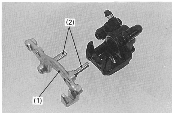
(1) キャリパスティ (2) ピンボルト
