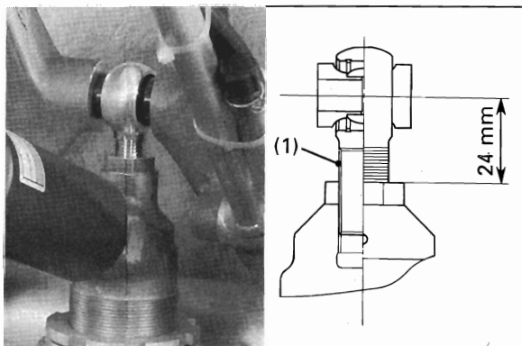
(1) アジャスタ
