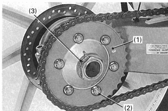
(1) ドリブスプロケット (2) ナット (3) ワイヤロック
