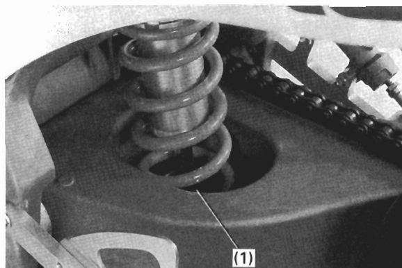
(1) O-リング
