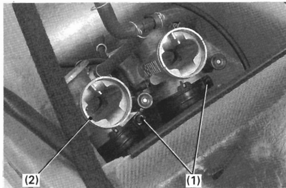
(1) バンドスクリュ (2) キャブレター
