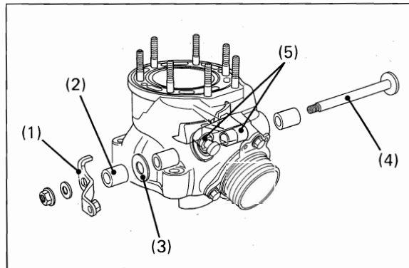
(1) バルブアーム (2) ディスタンスカラー (3) ワッシャ (4) フラップバルブシャフト (5) フラップバルブ
