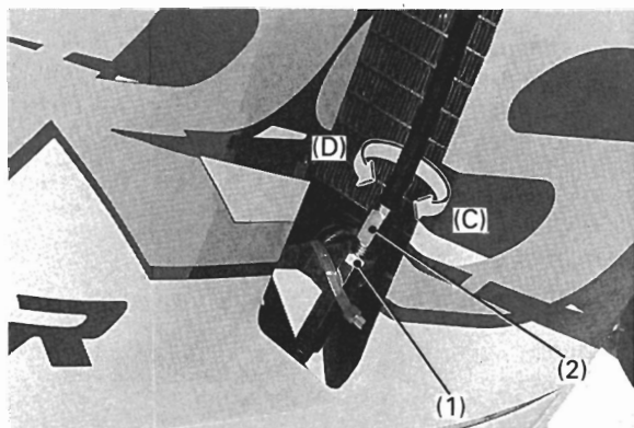
(1) ロックナット (2) アジャスタ
