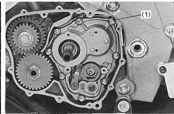
(1) ボルト
