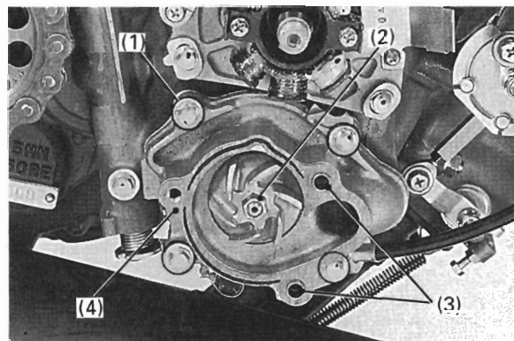
(1) ボルト (2) ワッシャ／インペラ (3) ノックピン (4) ガスケット
