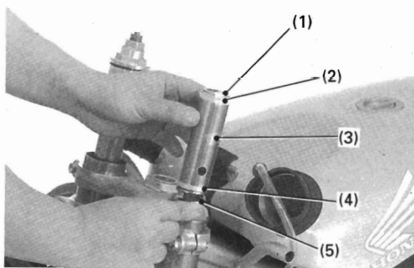
(1) スプリングシート (2) シートストッパ (3) スプリングカラー (4) ジョイントプレート (5) フォークスプリング
