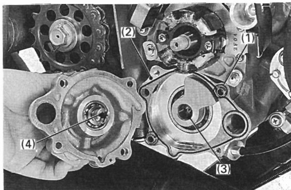
(1) ノックピン (2) ガスケット (3) 凸部 (4) 凹部
