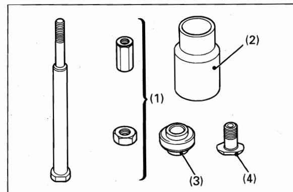
(1) ドライバシャフト Assy. (2) アッセンブリベース (3) アタッチメント (4) リム
