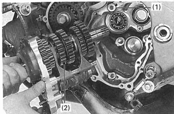
(1) ノックピン (2) トランスミッション/ホルダ Assy.
