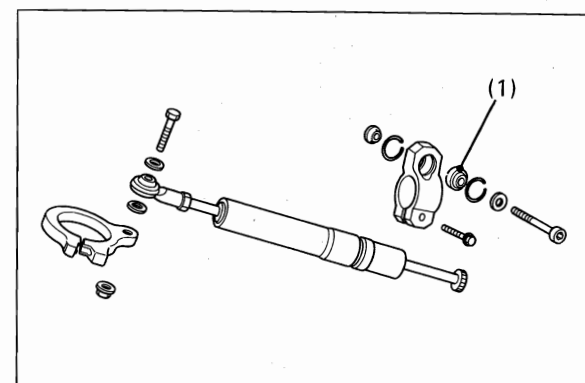
(1) スペリカルベアリング
