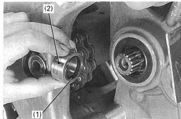
(1) オイルシール (2) カウンタシャフトカラー
