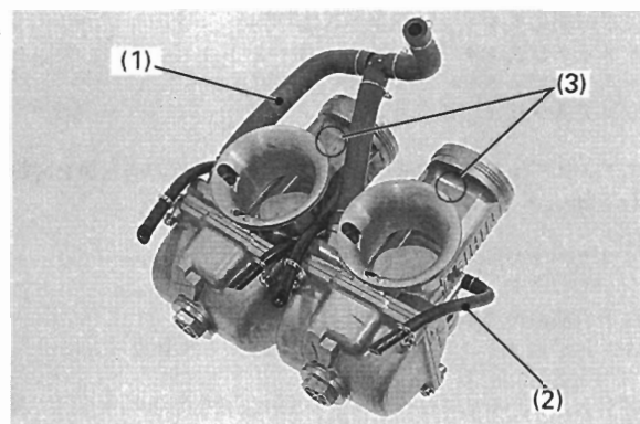
(1) フューエルチューブ (2) エアVENTチューブ (3) マーク
