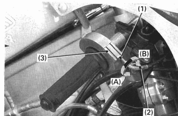
(1) ロックナット (2) スロットルケーブル (3) スロットルハウジング
